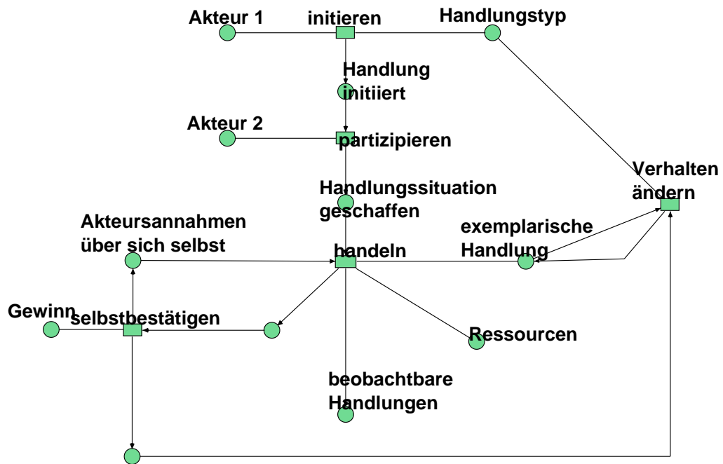
Abbildung 6: Handeln
