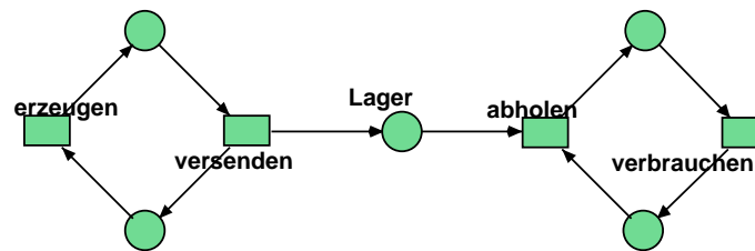
Abbildung 3: Erzeuger-Verbraucher Protokoll
