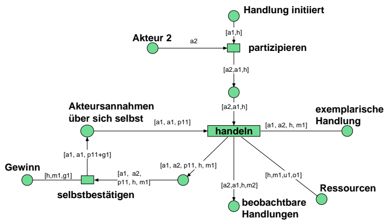
Abbildung 13: Protokoll: Angestellter
