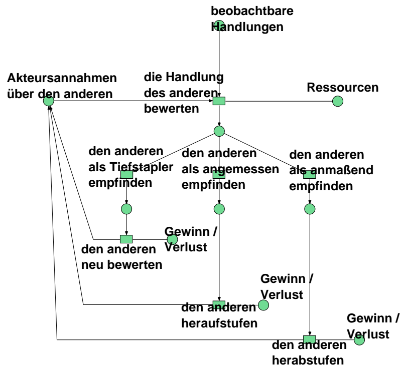
Abbildung 7: Wechselseitig bewerten
