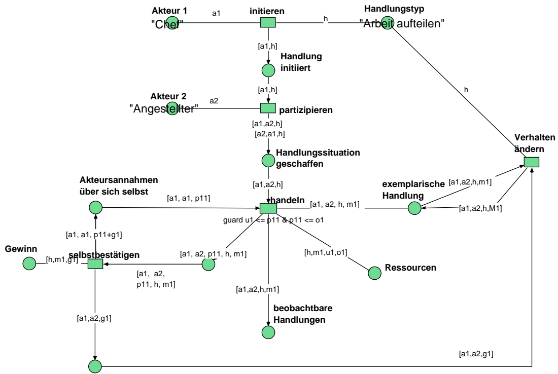
Abbildung 9: Handeln
