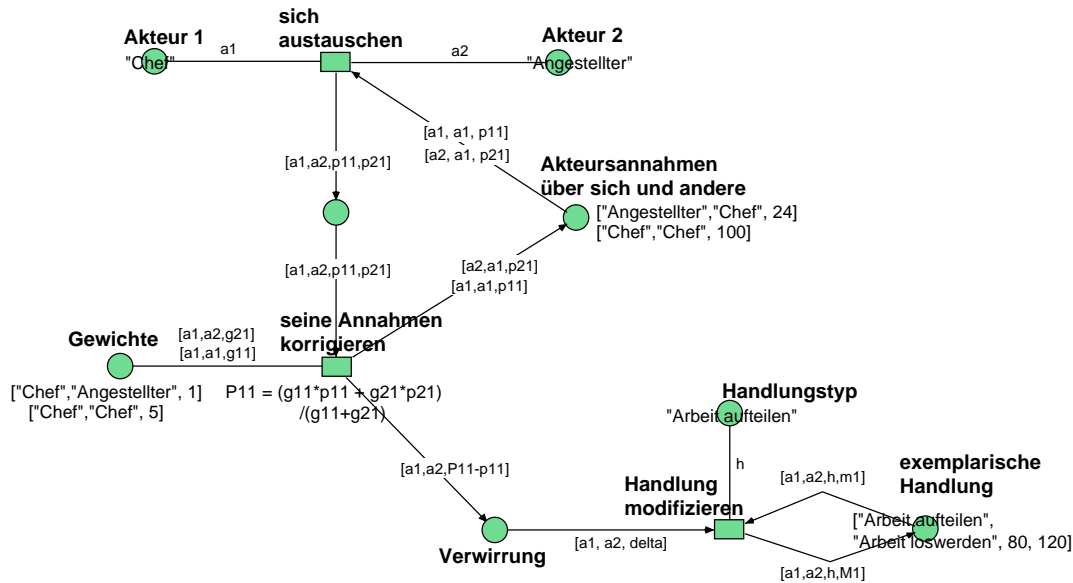
Abbildung 11: Anpassungshandlungen
