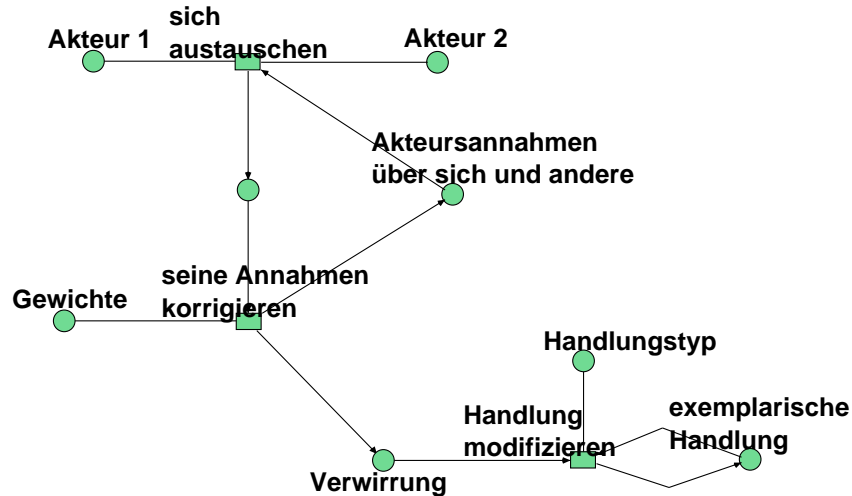
Abbildung 8: Handlungsanpassung
