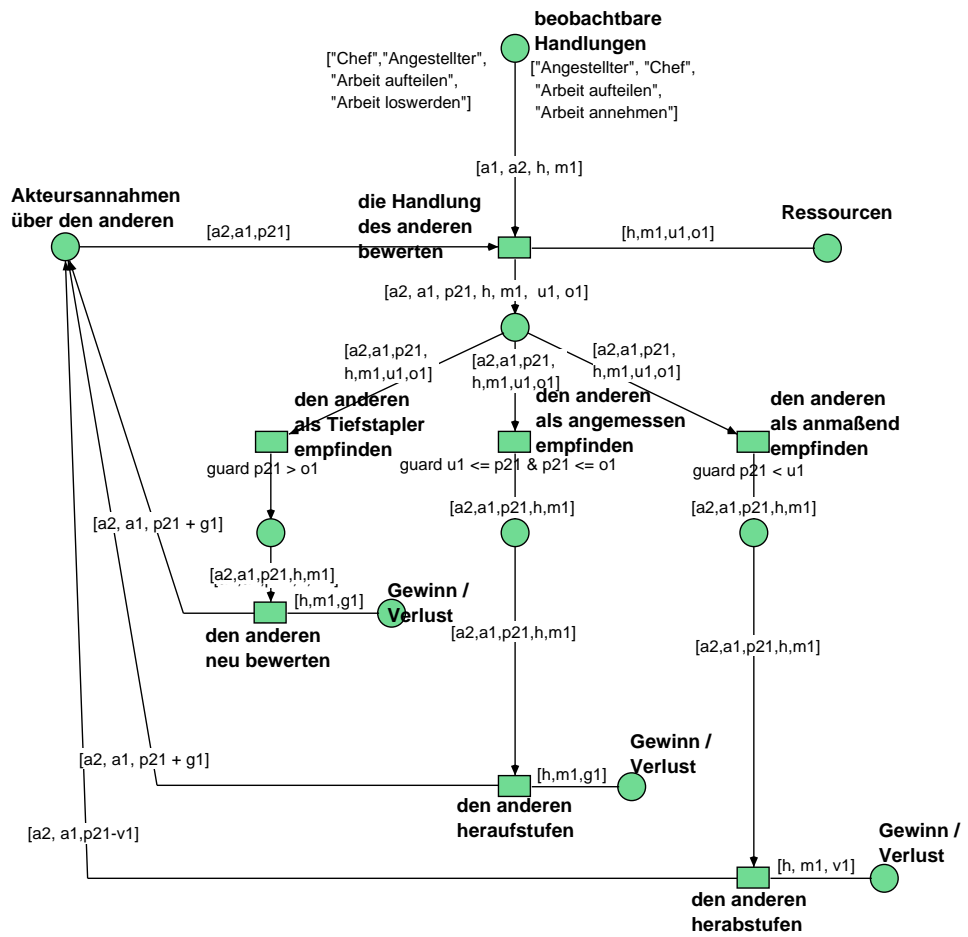
Abbildung 10: Wechselseitige Bewertung
