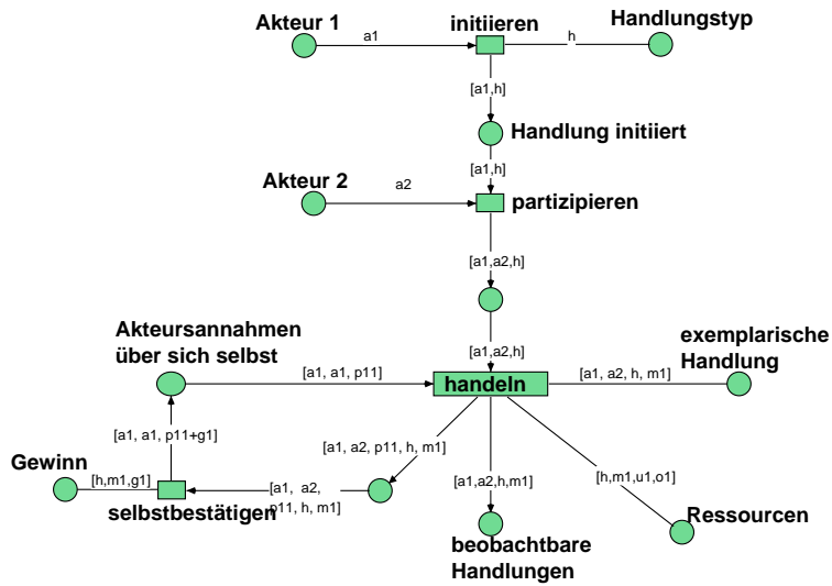
Abbildung 12: Protokoll: Chef
